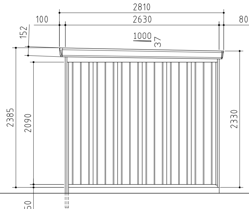
側面図
